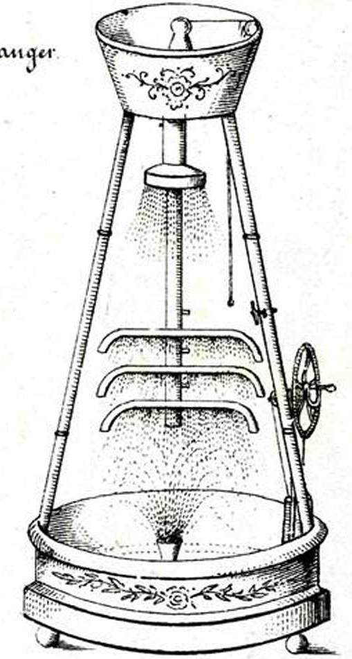
Appareil pour douches en pluie.
